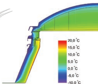
Izotermický děj JET TOP-90 Plus
